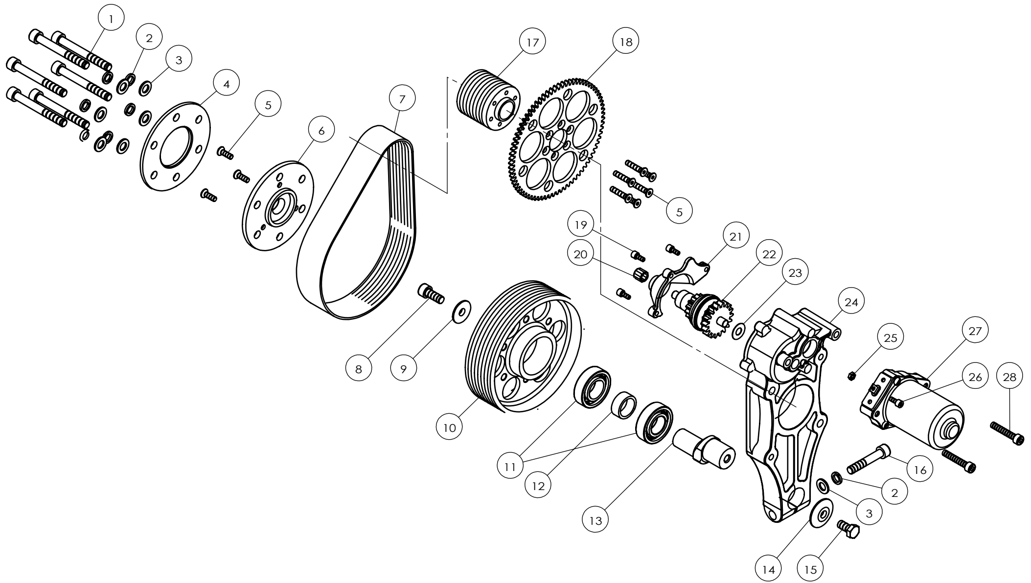
DLE200-----减速部分 Reduction Part
