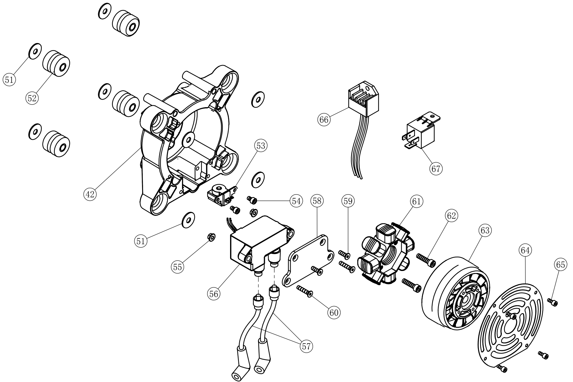
DLE200——点火部分 Ignition Part
