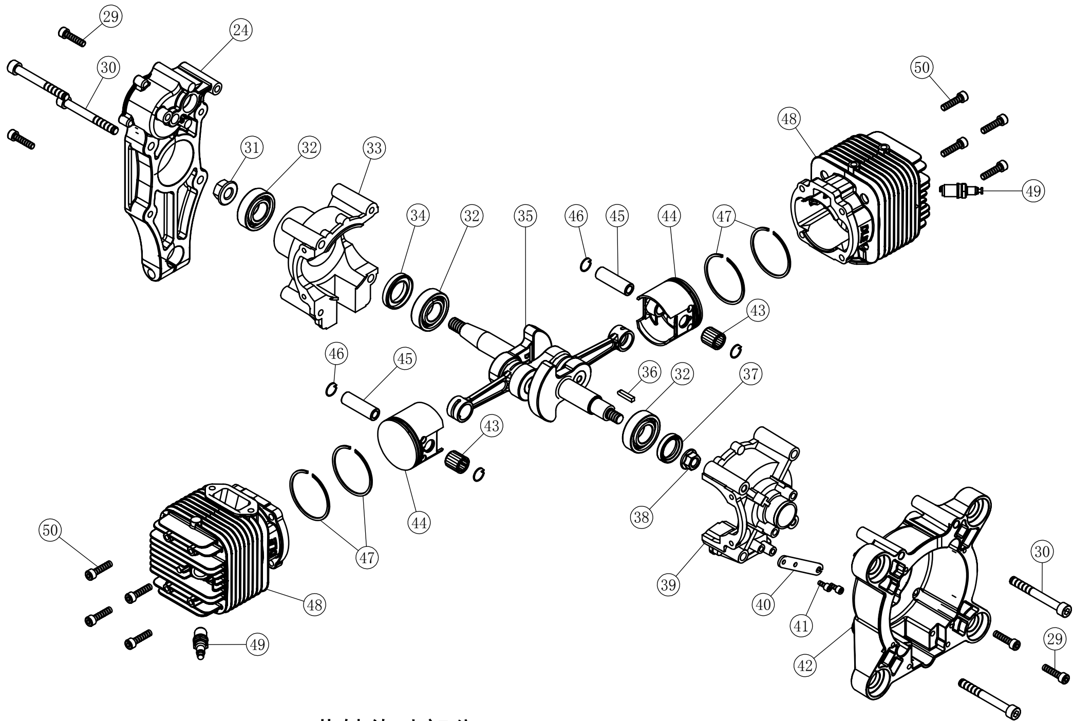
DLE200-----曲轴传动部分 Crankshaft Drive Part
